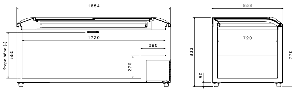
Kopfgerät PARIS 185
