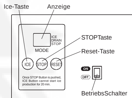
Bedienungstafel
