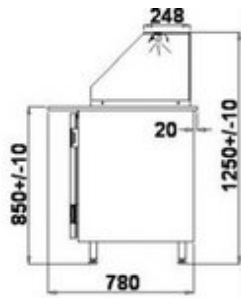
730155-205-255-u- 731105-155 Seitenskizze2
