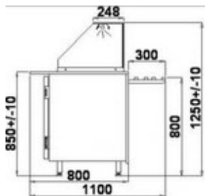
730155-205-255-u- 731105-155 Seitenskizze
