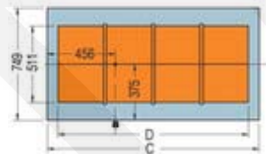
Armonia2bis6-Bain-Marie-Draufsichtsskizze
