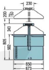
Seitenskizze Stille Kühlung
