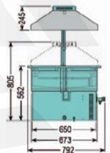
Seitenskizze Umluftkühlung
