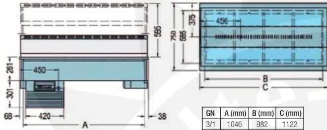
Vermaßungsskizze Stille Kühlung
