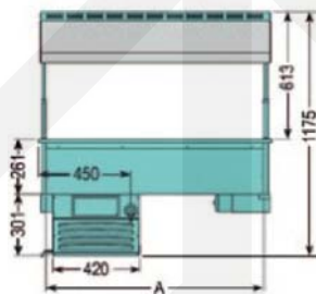
Vermaßungsskizze Umluftkühlung
