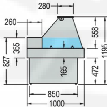
Oceanus Seitenskizze
