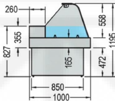
Oceanus C-Seitenskizze
