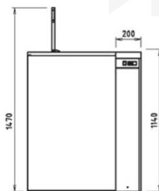
Frontskizze NMK 240 ZK
