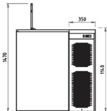
Frontskizze NMK 240
