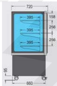
23120005-Seitenskizze
