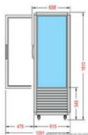
23301383- Seitenskizze
