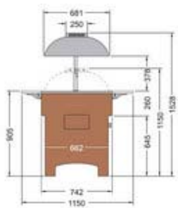
23500080-81-82- Seitenskizze
