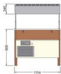
23500080- Frontskizze
