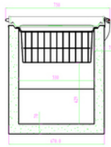
915034 915035 Seitenskizze
