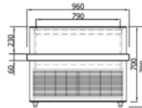
309750 Seitenskizze
