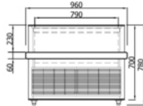
309900 Seitenskizze
