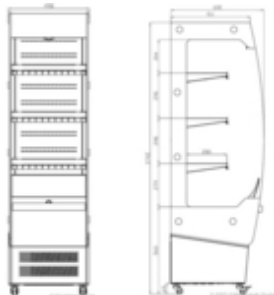
Frontskizze Seitenskizze
