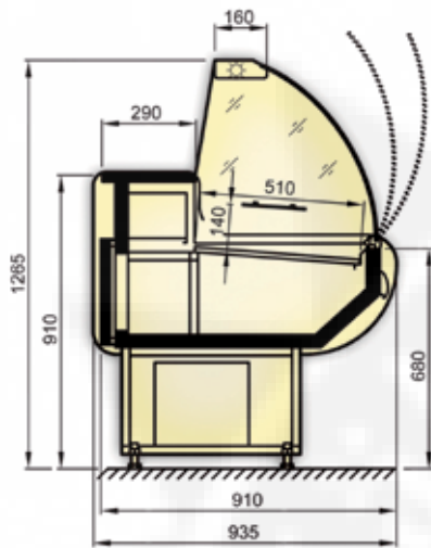
Maßzeichnung
