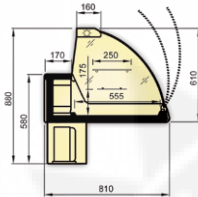
Maßzeichnung
