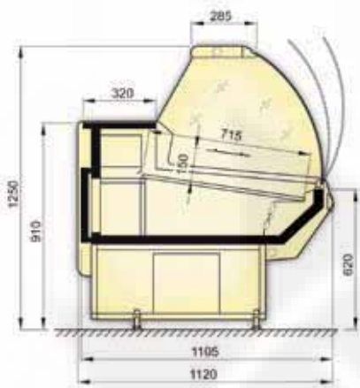
Maßzeichnung
