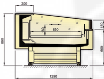
Lhotse 09 LDL-OM-SB Maßzeichnung SB-Variante
