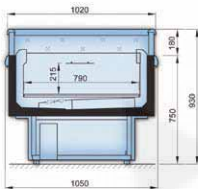
Maßzeichnung
