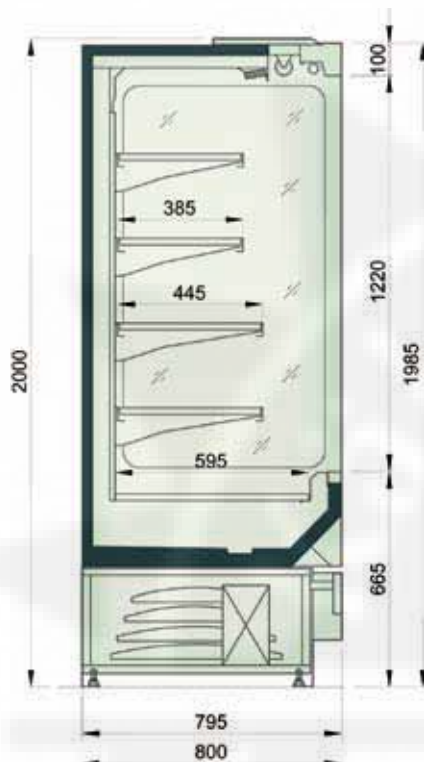
Maßzeichnung
