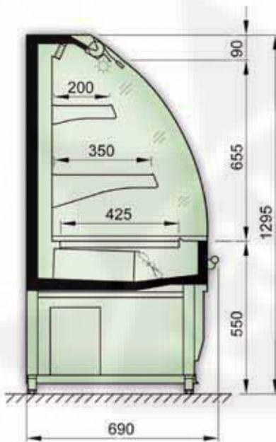
Maßzeichnung
