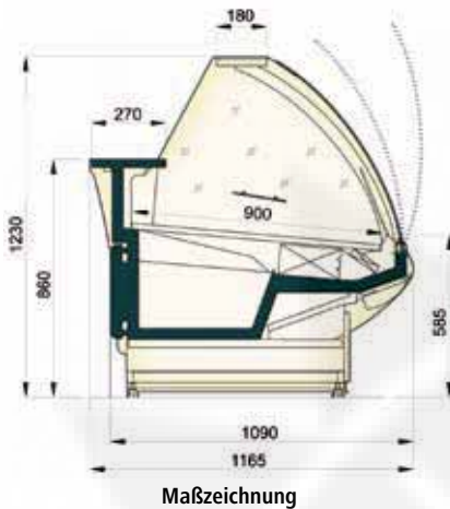
Maßzeichnung
