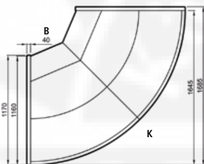
Grazia 04 LDG-OM NZ 90 Maßzeichnung
