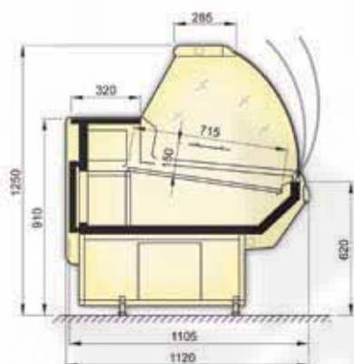
Maßzeichnung
