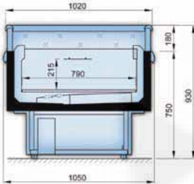
Maßzeichnung
