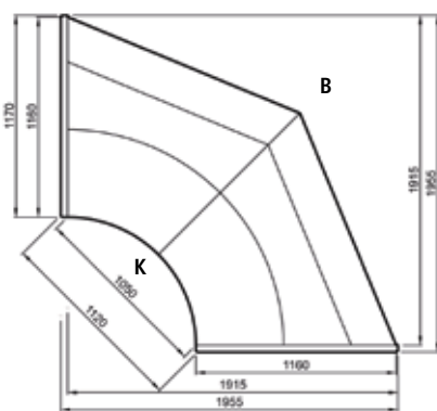
Grazia 04 LDG-OM NW 90 Maßzeichnung
