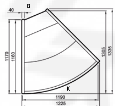
Grazia 04 LDG-OM NZ 45 Maßzeichnung
