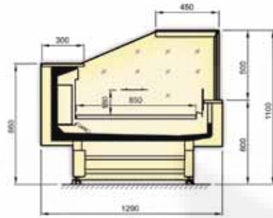
Maßzeichnung
