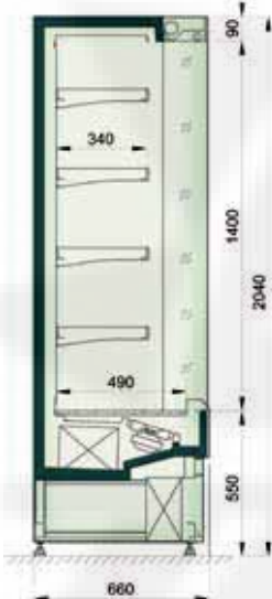
Maßzeichnung
