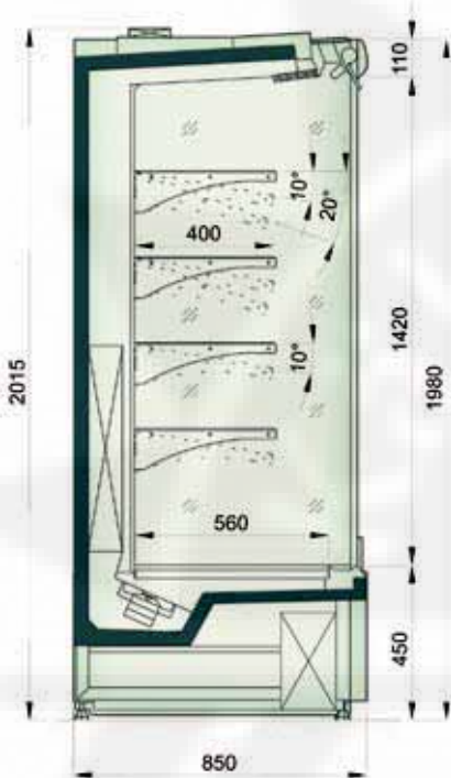
Maßzeichnung
