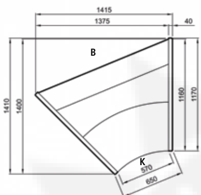
Grazia 04 LDG-OM NW 45 Maßzeichnung
