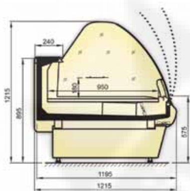
Maßzeichnung
