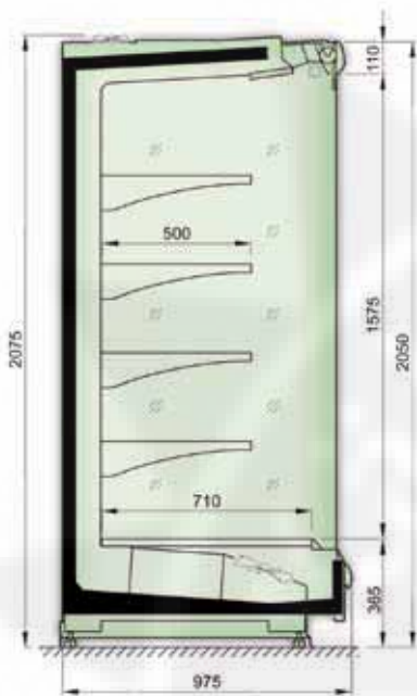
Maßzeichnung
