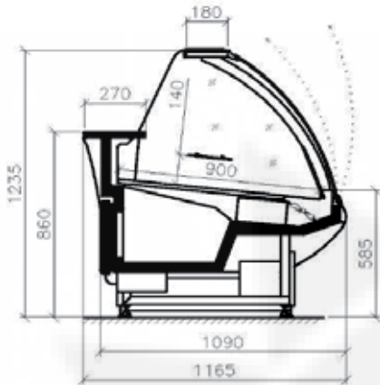
Maßzeichnung
