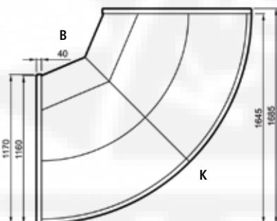
Grazia 04 LDG-OM NZ 90 Maßzeichnung
