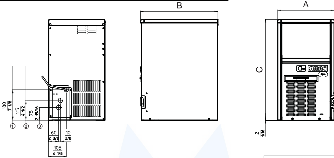
SDN 25 - 30
