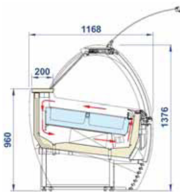
Maßzeichnung
