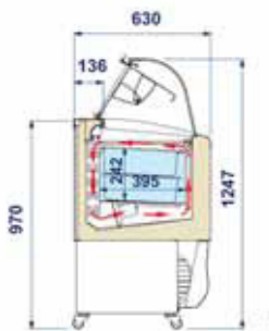
Maßzeichnung FIJI 4,6,7,9,12
