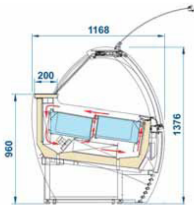
Maßzeichnung
