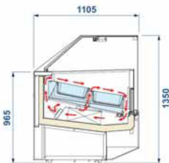
Maßzeichnung
