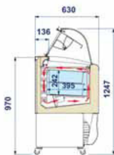
Maßzeichnung SAMOA 4,6,7,9,12
