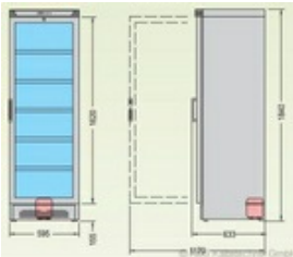
Frontund Seitenskizze
