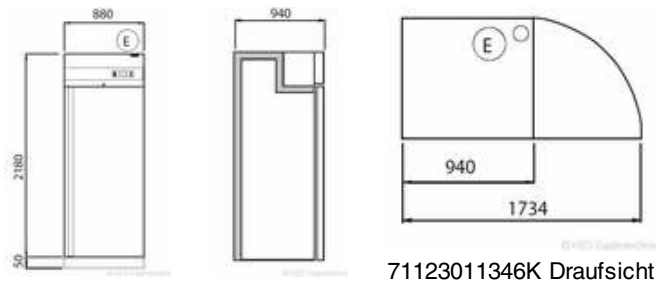
71123011346K Frontansicht
