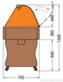
23500003ND Seitenansicht
