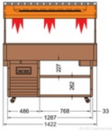
23500003ND Frontansicht
