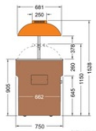
23500090-91-92- Seitenkizze
