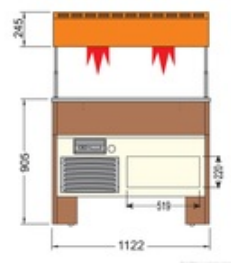
23500090- Frontskizze
