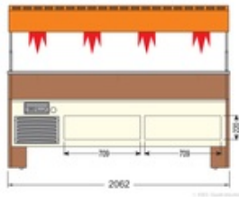
23500092-Frontskizze
