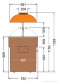
23500090-91-92- Seitenkizze
