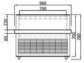
309114 Seitenskizze
