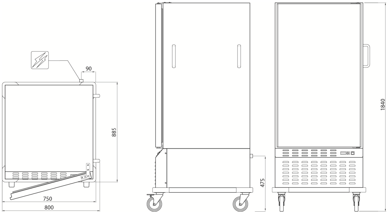
Model HCT 132E (type HCT 132E) - Model HFT 132E (type HFT 132E)
