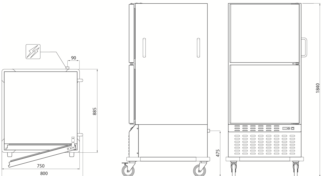
Model HCT 102E (type HCT 102E) - Model HFT 102E (type HFT 102E)
