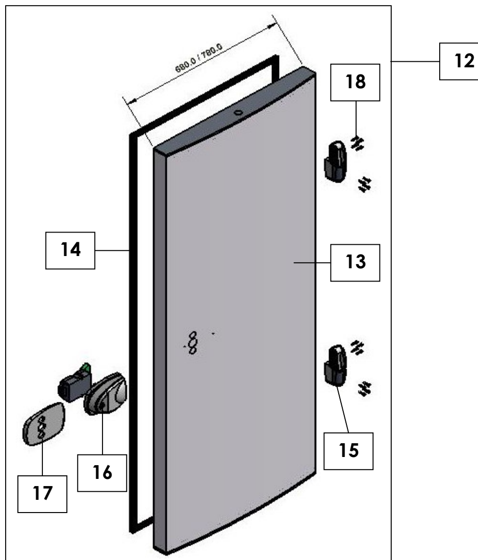
PANELS OF THE FRAME AND DOORS / PANNEAUX DU CERCEAU ET DES PORTES / WÄNDE DES RAHMENS UND DER TÜR
