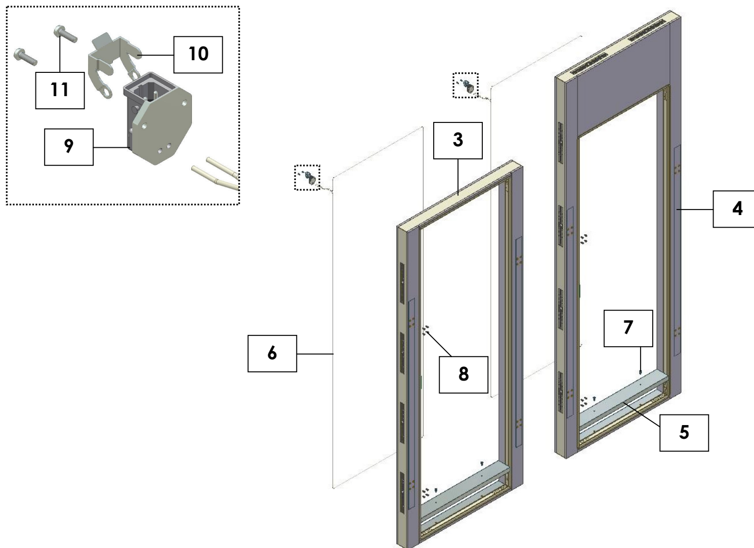
PANELS OF THE FRAME AND DOORS / PANNEAUX DU CERCEAU ET DES PORTES / WÄNDE DES RAHMENS UND DER TÜR
