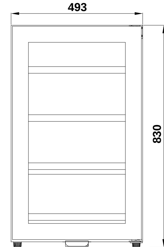
Vorderansicht
