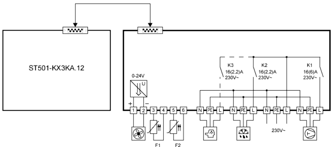
Abbildung 1: Anschlußbelegung
