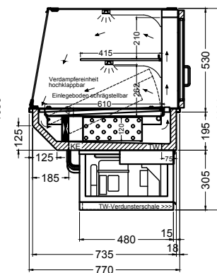
BAK GS-132-53-E
