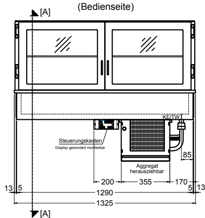
(Bedienseite)
