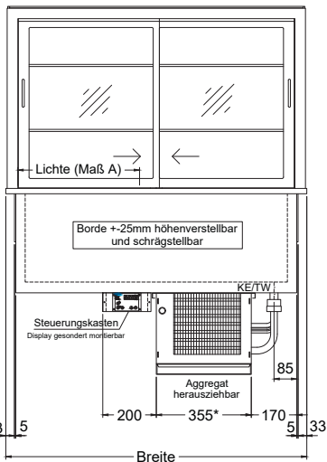
(Bedienseite)
