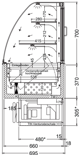
(Schnitt > rund)
