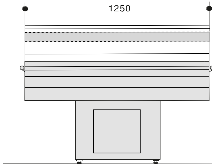
Vorderansicht
