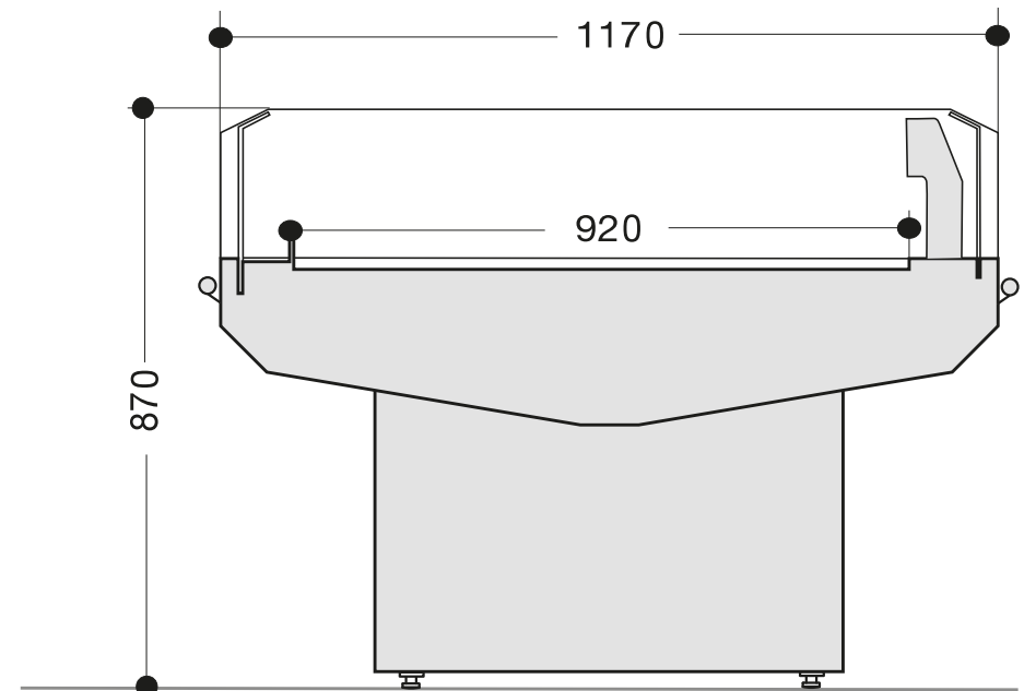
Seitenansicht
