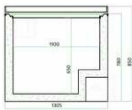
916039 Frontskizze
