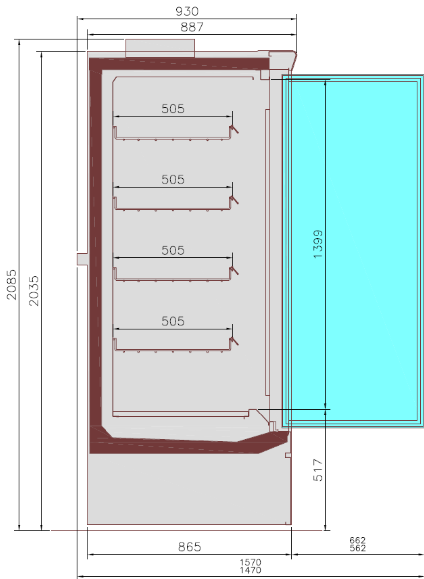
Código: C279106A1 Medidas: mm Escala: 1:10 Designação: CORTE COMERCIAL BARTOLOMEU BT (PORTA ABERTA)
