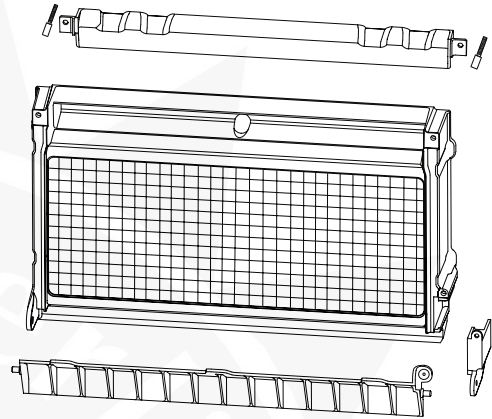
Die Daumenschraube vom Behälterschalterdeckel entfernen – dabei die Klappe abstützen, und dann entfernen
