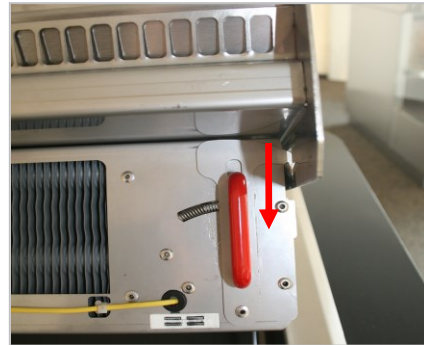
Abb. 6.21 Beidseitig die roten Griffe nach unten schieben (sichern).
