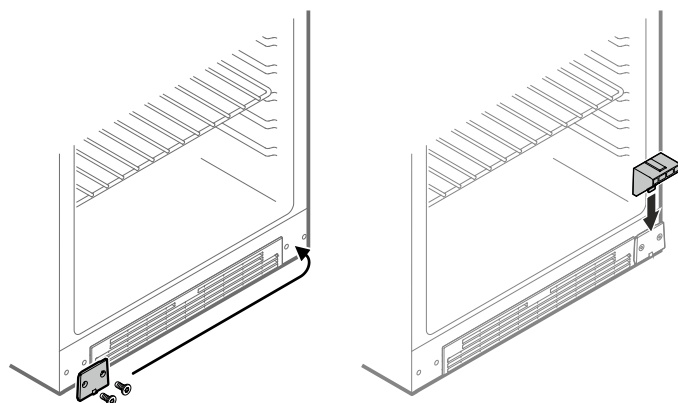
20. Transportsicherung aufsetzen.
