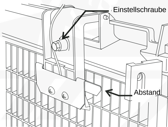
Eis thickness Justage des Sensors
