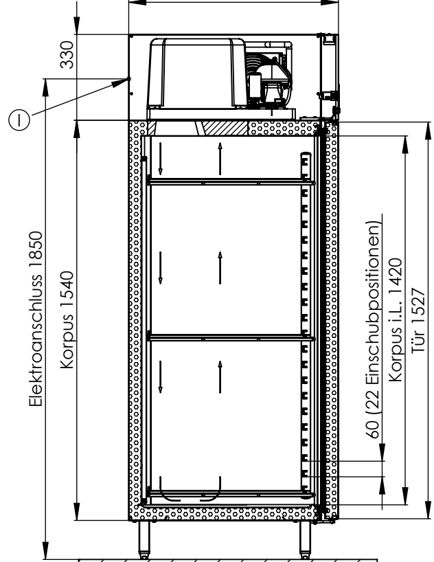
SCHNITT A-A
