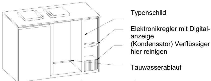
Bild 3: Draufsicht Abfallkühler, Eigenkühlung, steckerfertig
