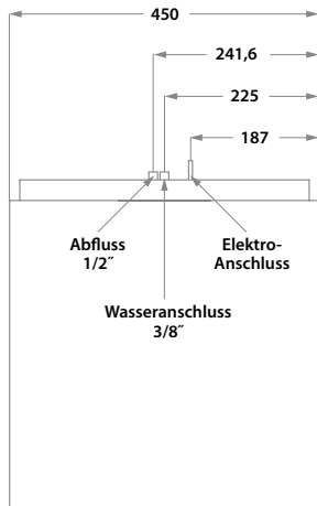
Draufsicht
