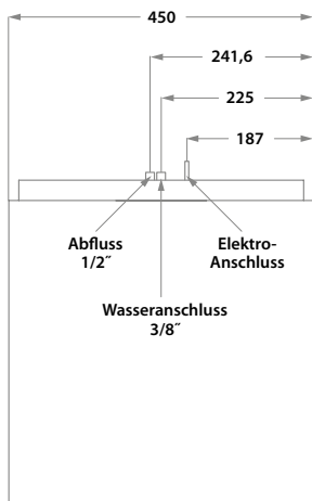
Draufsicht
