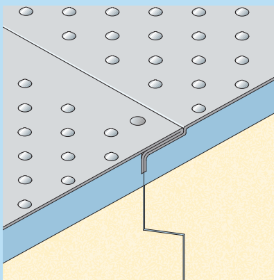
Edelstahlboden, kegelverpresst
