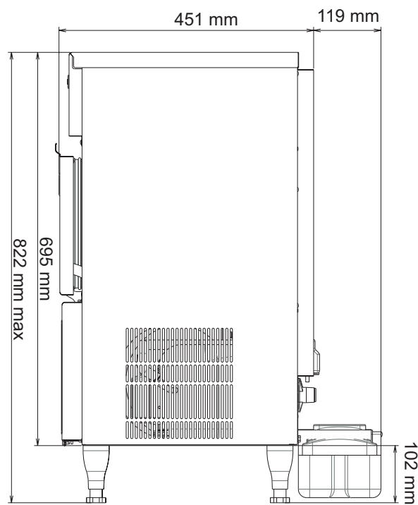
PUMPE AN DER RÜCKSEITE
