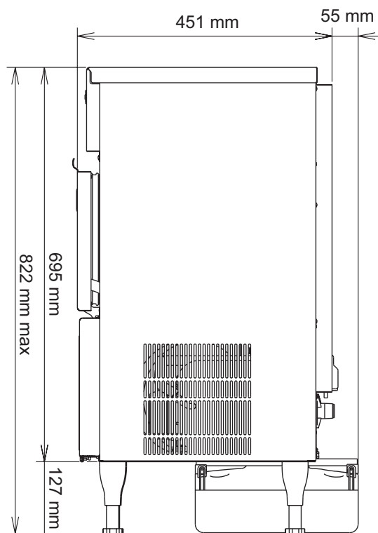
PUMPE UNTER DEM GERÄT
