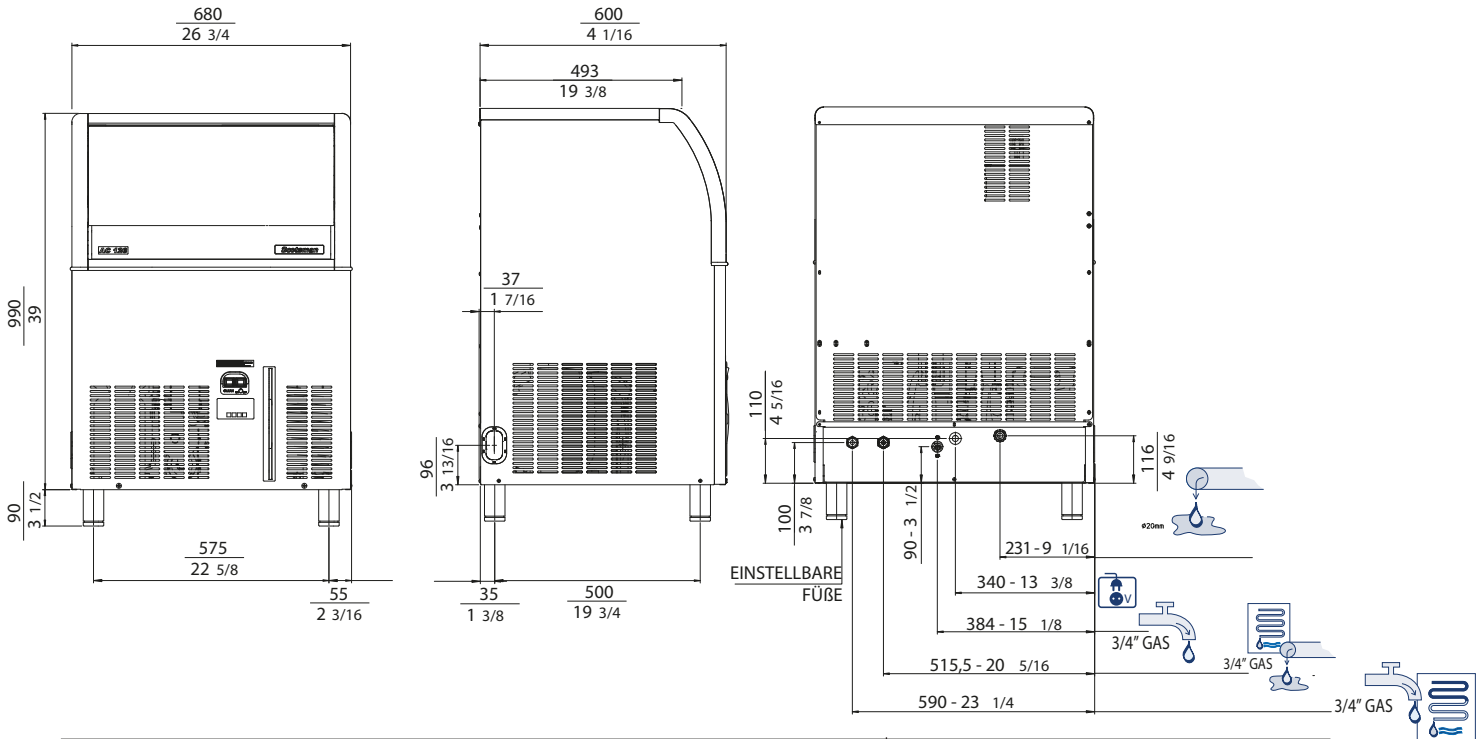
AC 176 LUFTEGKÜHLT
