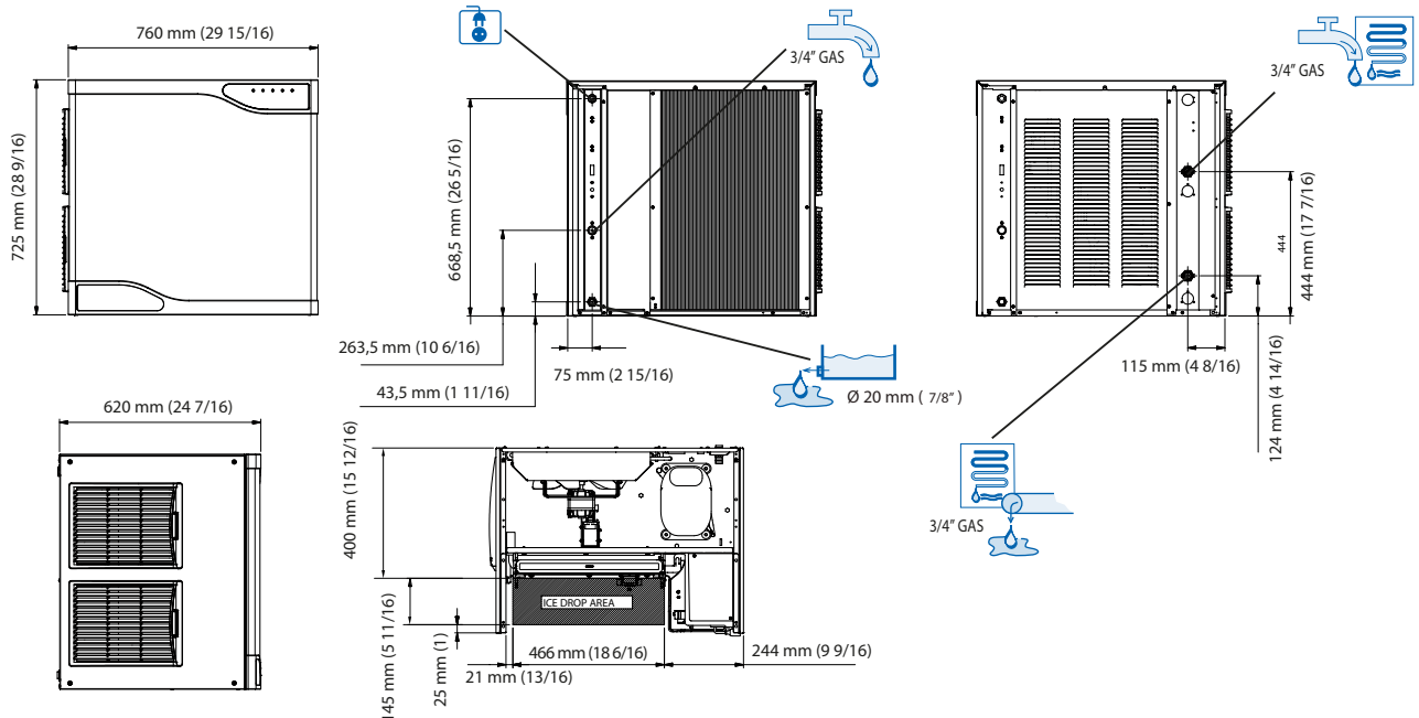
MV1006 LUFTGEKÜHLT
