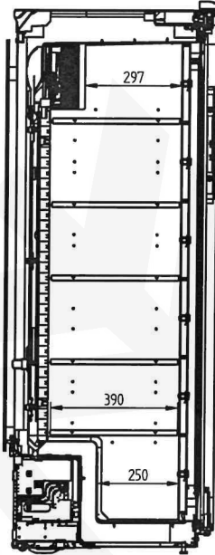
Schnitt A-A
