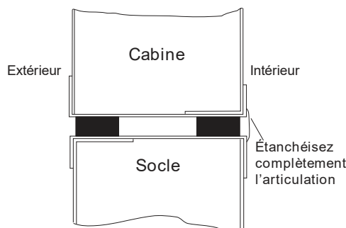
Coupe transversale de la cabine et du socle
