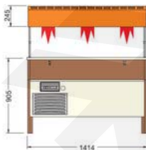
23500091-Frontskizze
