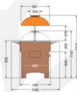
23500090-91-92- Seitenkizze
