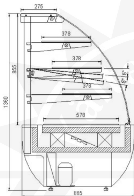
Holzgehäuse
