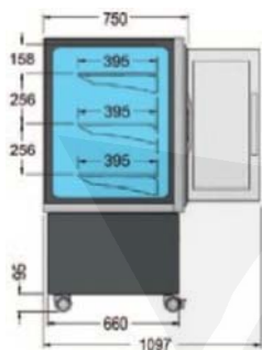
Seitenskizze zu Karina 96
