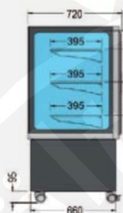
Seitenskizze zu Karina 136 und Karina 186
