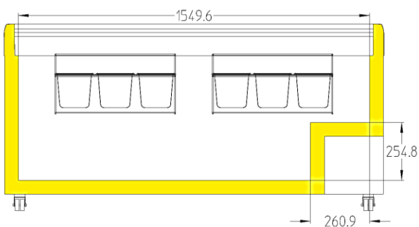
EFI 48.. / EFE51..
