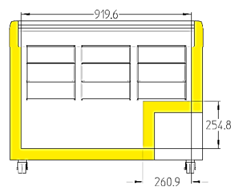
EFI 28.. / EFE 30..
