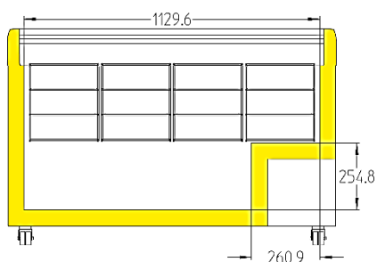
EFI 35.. / EFE 38..
