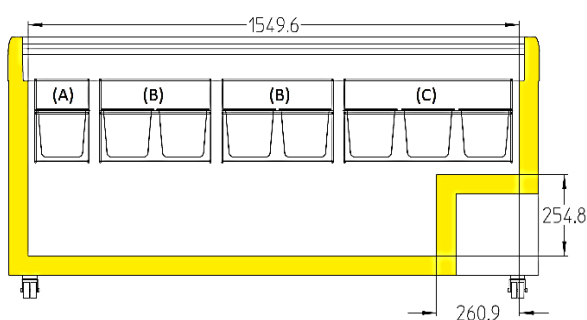
EFI 48.. / EFE51..
