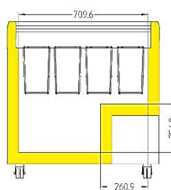
EFI 21.. / EFE22..
