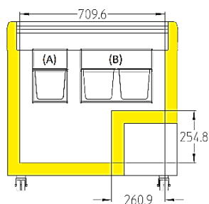
EFI 21.. / EFE22..
