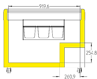
EFI 28.. / EFE 30..
