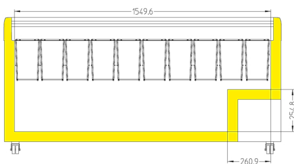
EFI 48.. / EFE51..
