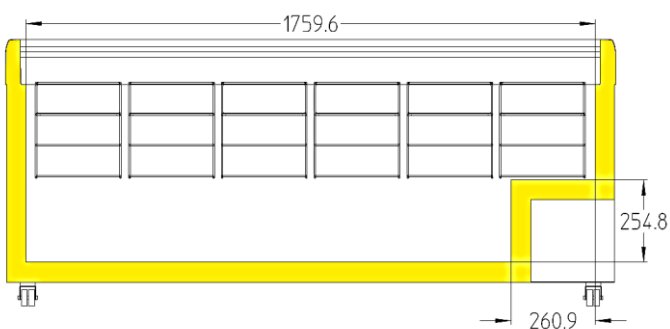
EFI 56.. / EFE60..
