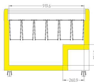
EFI 28.. / EFE 30..
