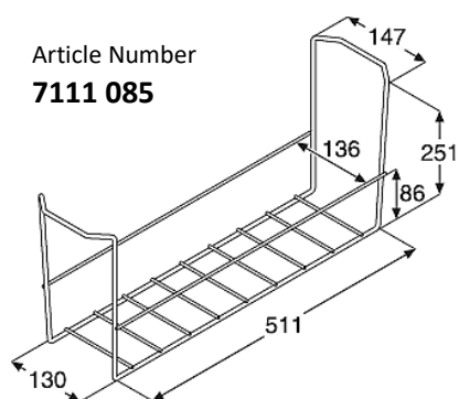
EFI 14.. / EFE15..
