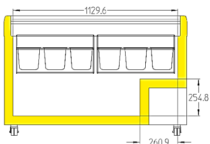
EFI 35.. / EFE 38..
