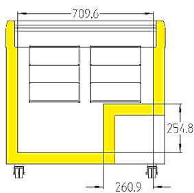
EFI 21.. / EFE22..
