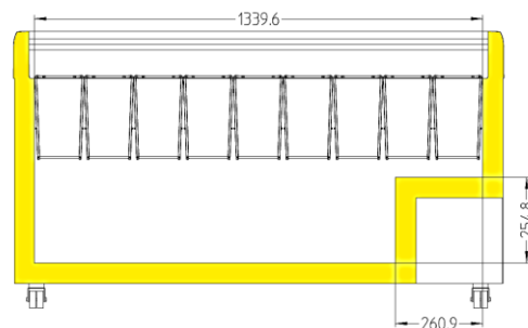
EFI 44.. / EFE 46..
