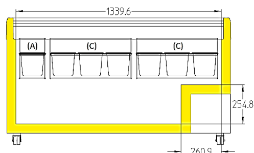
EFI 44.. / EFE 46..
