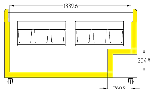
EFI 44.. / EFE 46..
