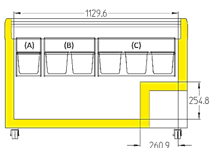
EFI 35.. / EFE 38..
