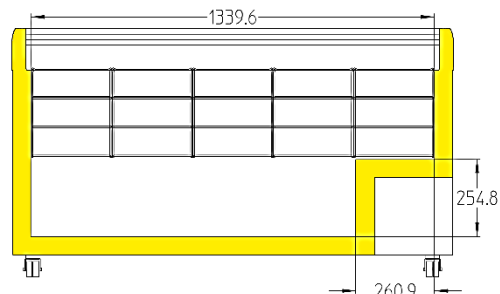
EFI 44.. / EFE 46..
