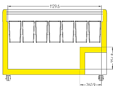
EFI 35.. / EFE38..
