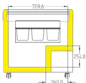
EFI 21.. / EFE22..
